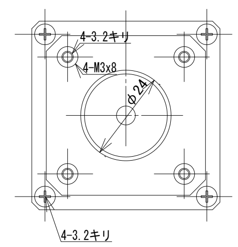
BB視図
